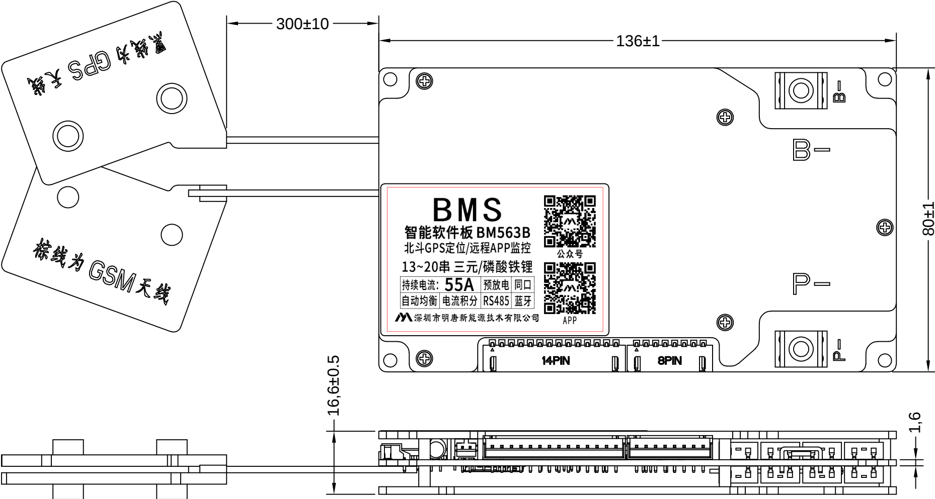
BM563B整机示意图
