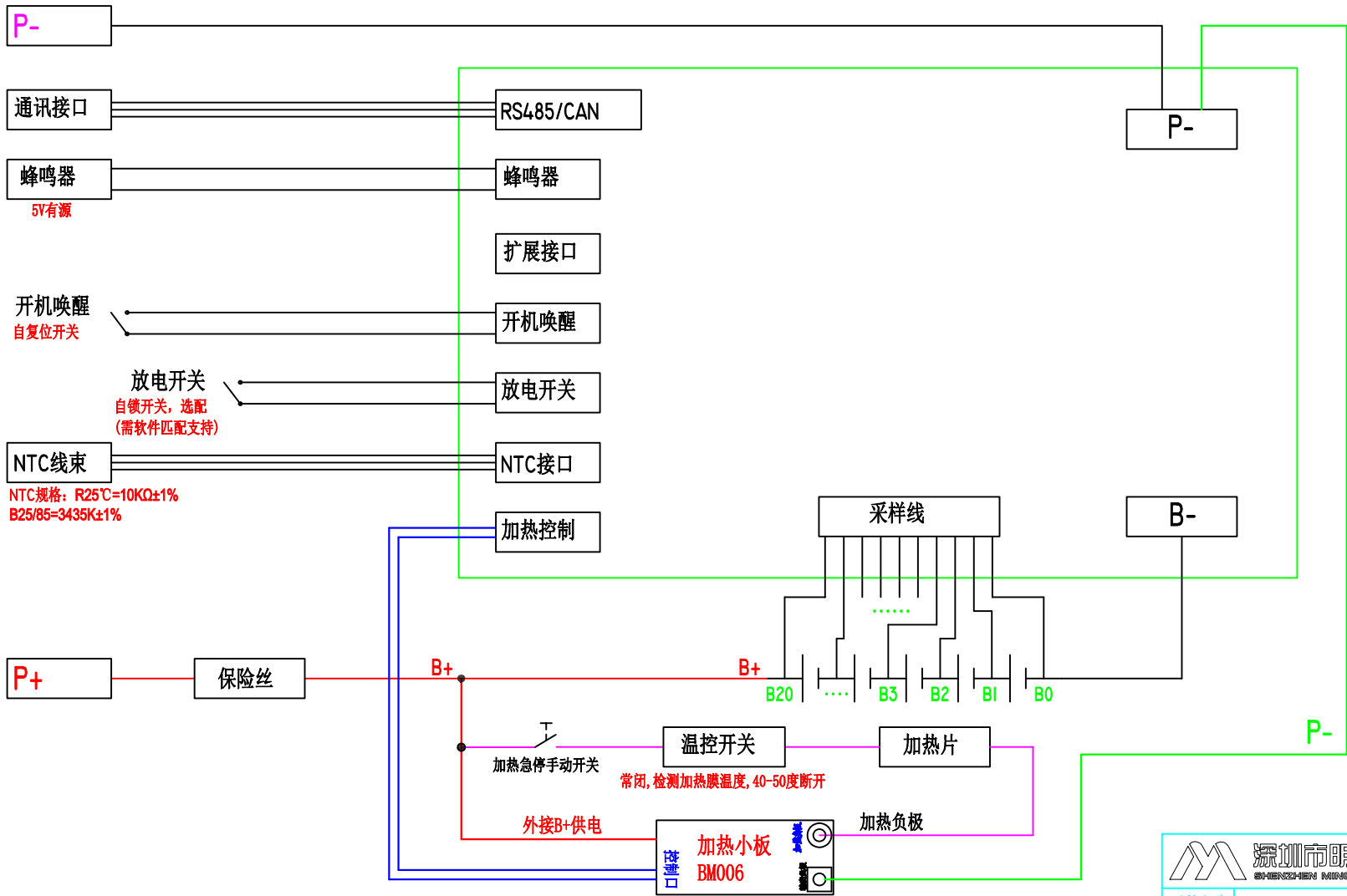
BM560-接线示意图
