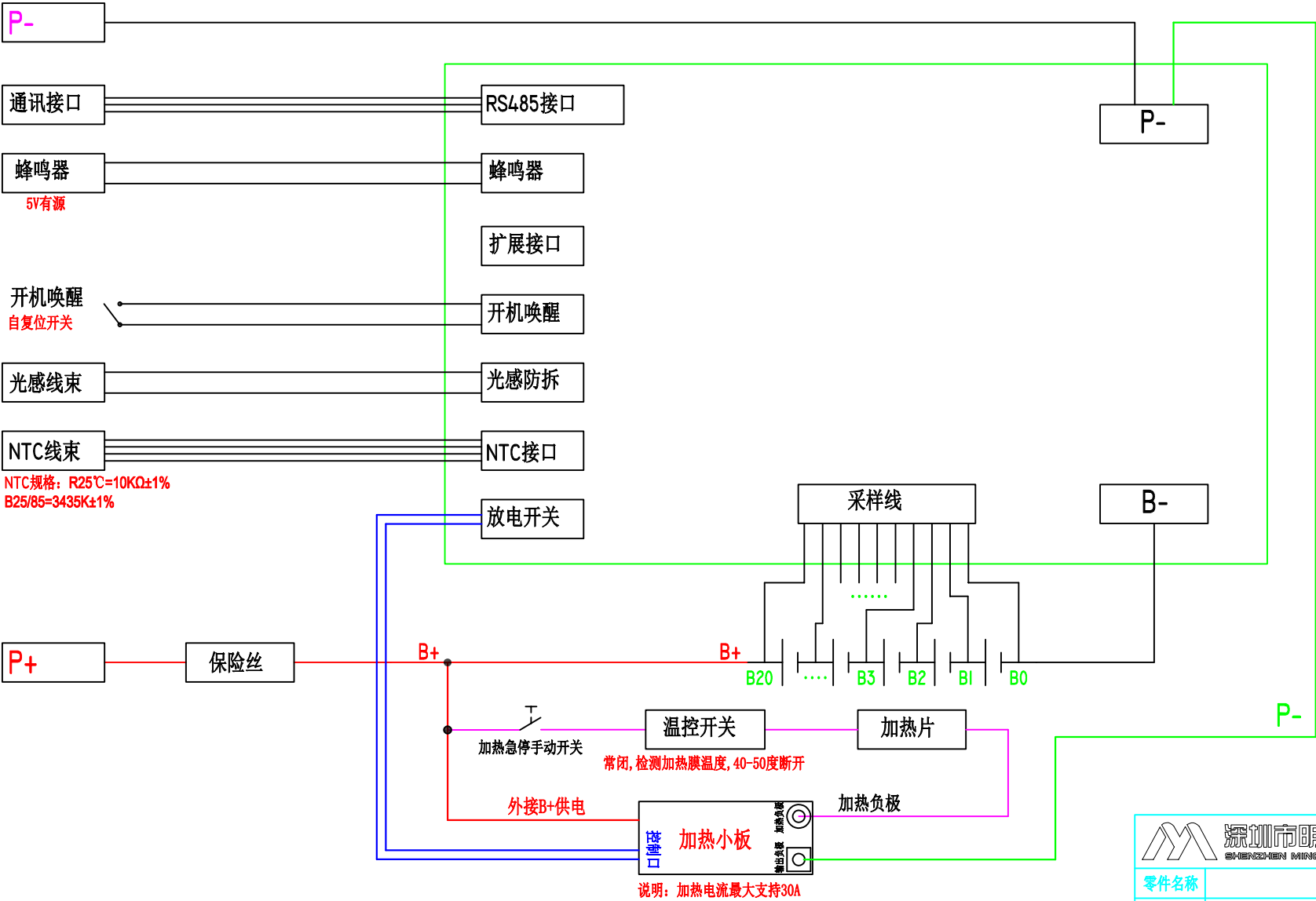
BM561C-接线示意图
