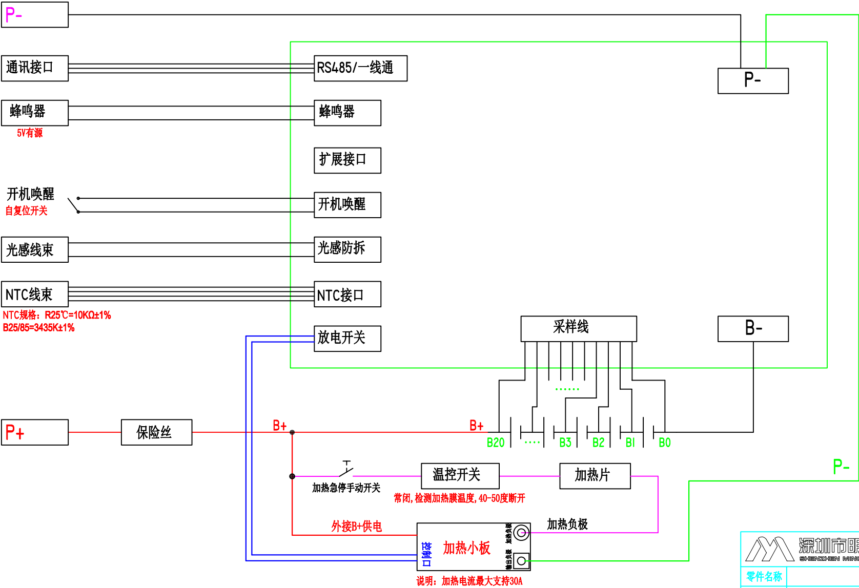
BM326-接线示意图
