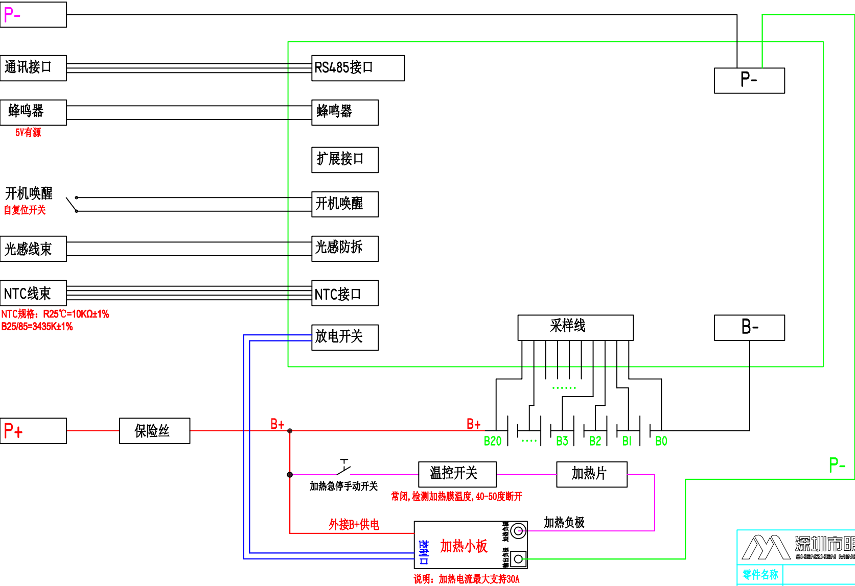
BM327-接线示意图
