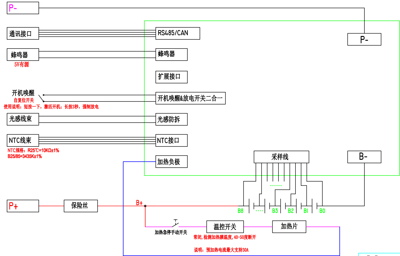
BM576A-接线示意图
