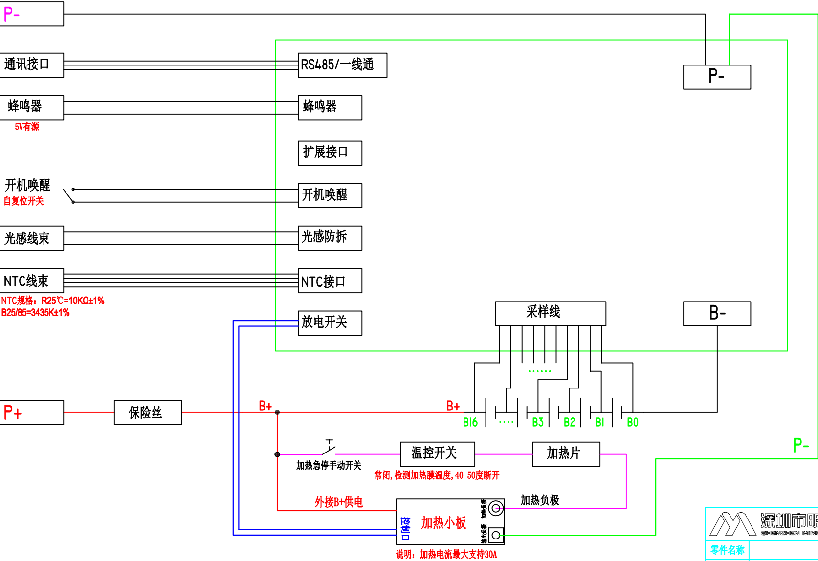
BM705-接线示意图
