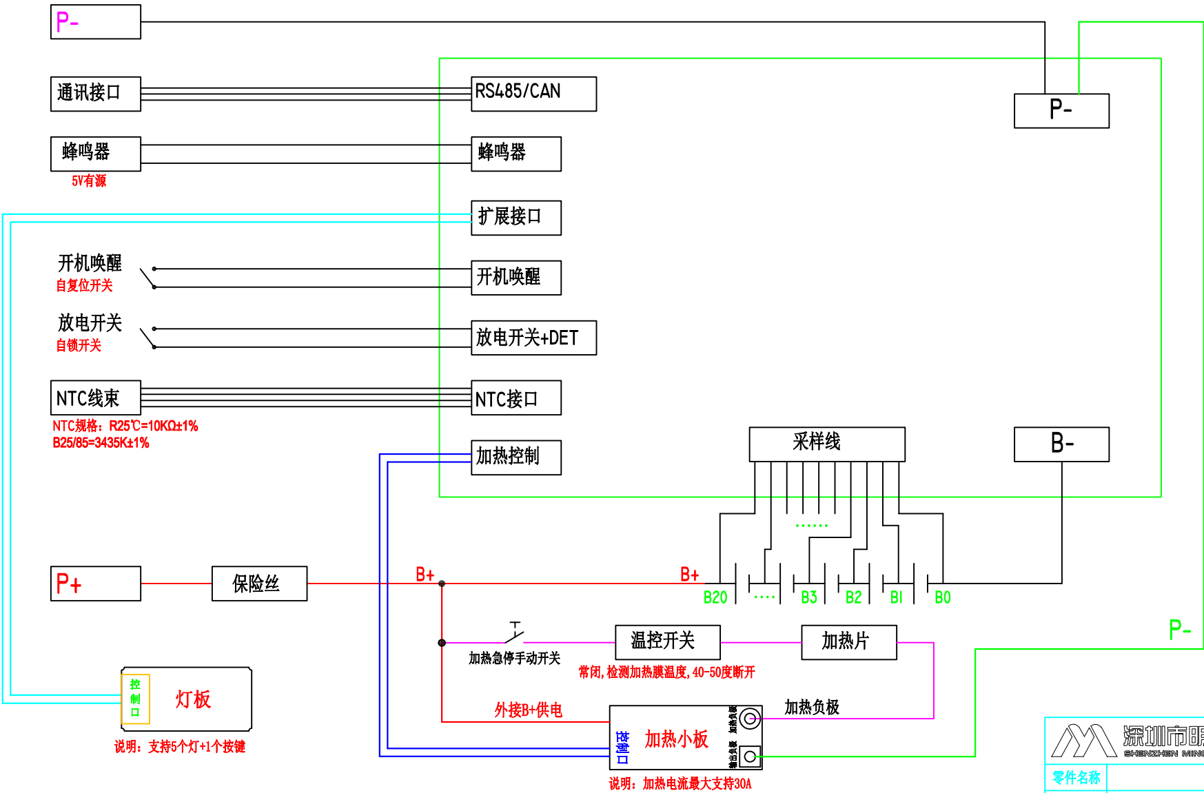
BT101-接线示意图
