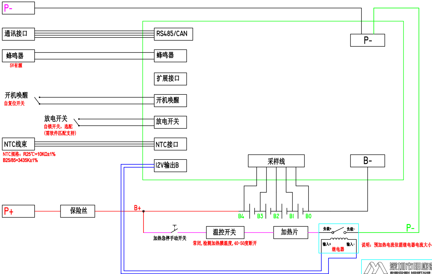
BM210-接线示意图
